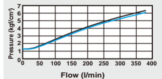
Model: SA530-01D
